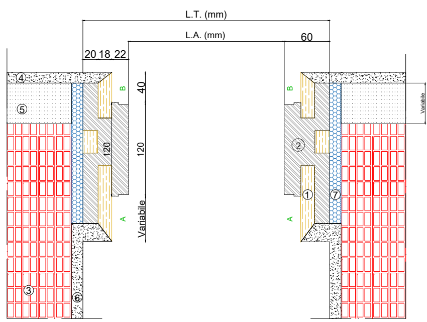
Sezione orizzontale
