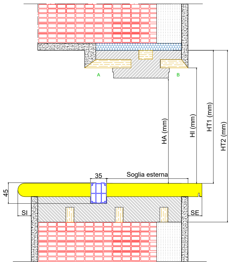
Sezione verticale
