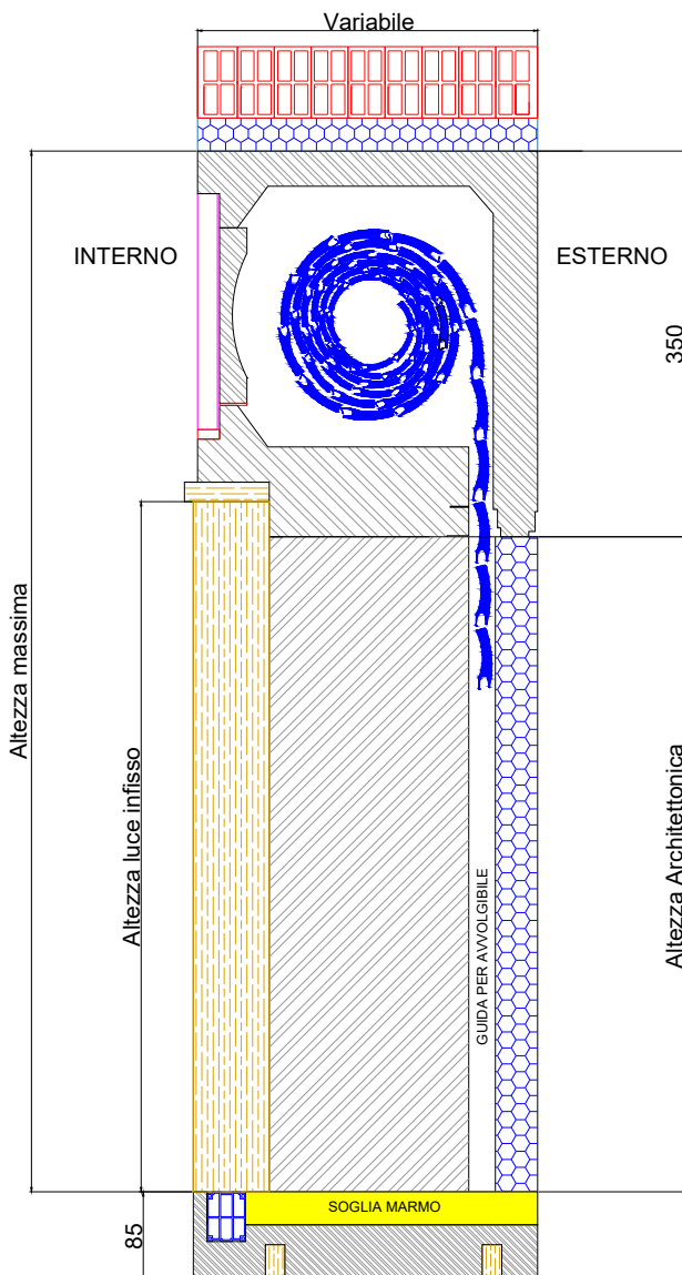
Sezione laterale
