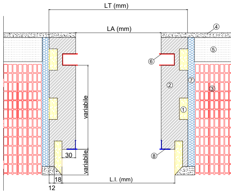
Sezione orizzontale
