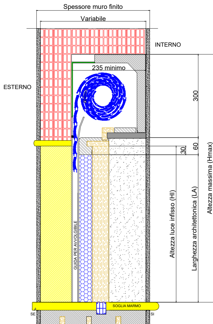
Sezione laterale
