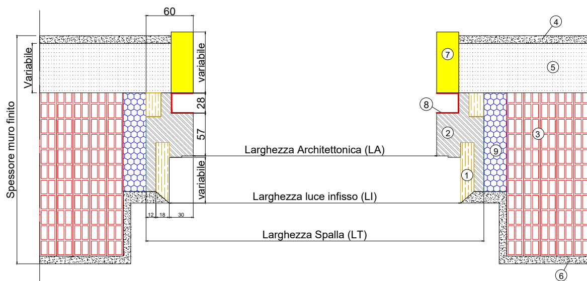
Sezione orizzontale
