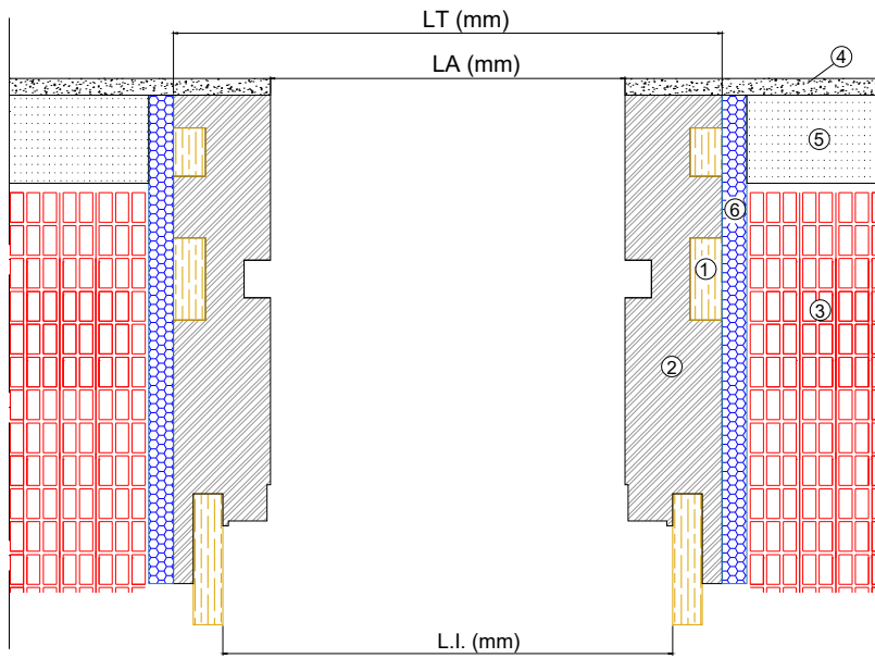
Sezione orizzontale
