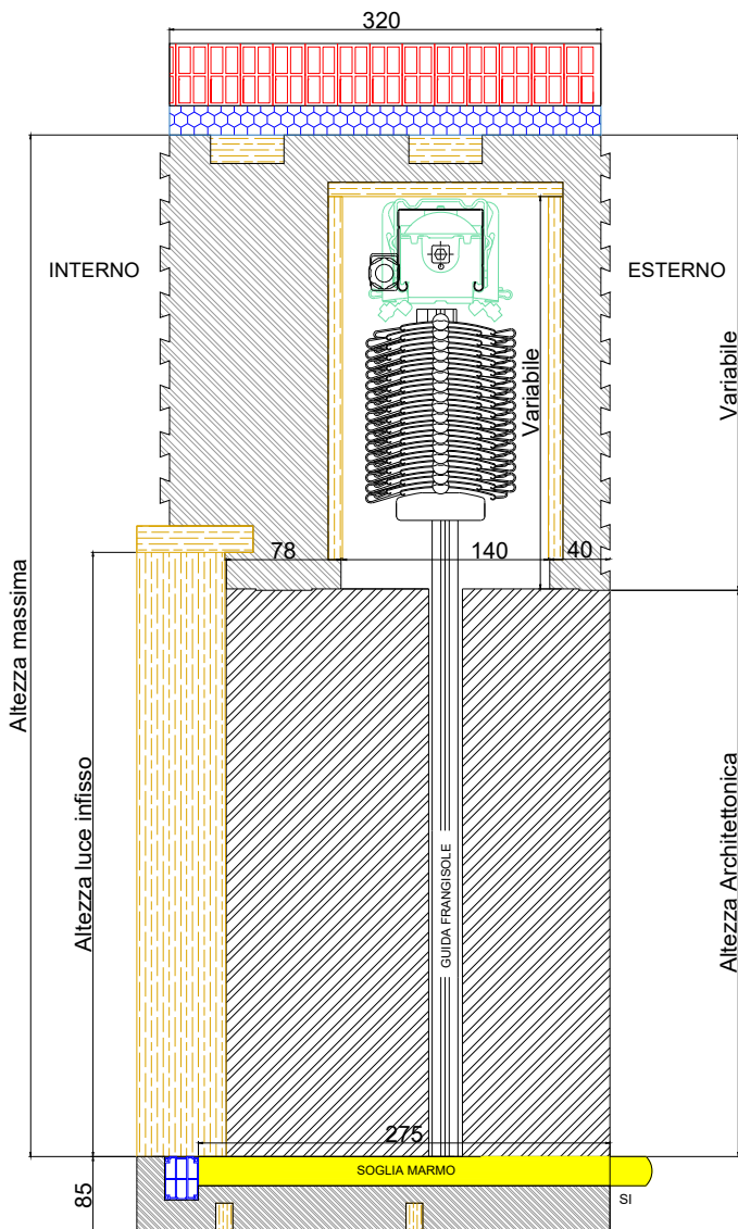
Sezione laterale
