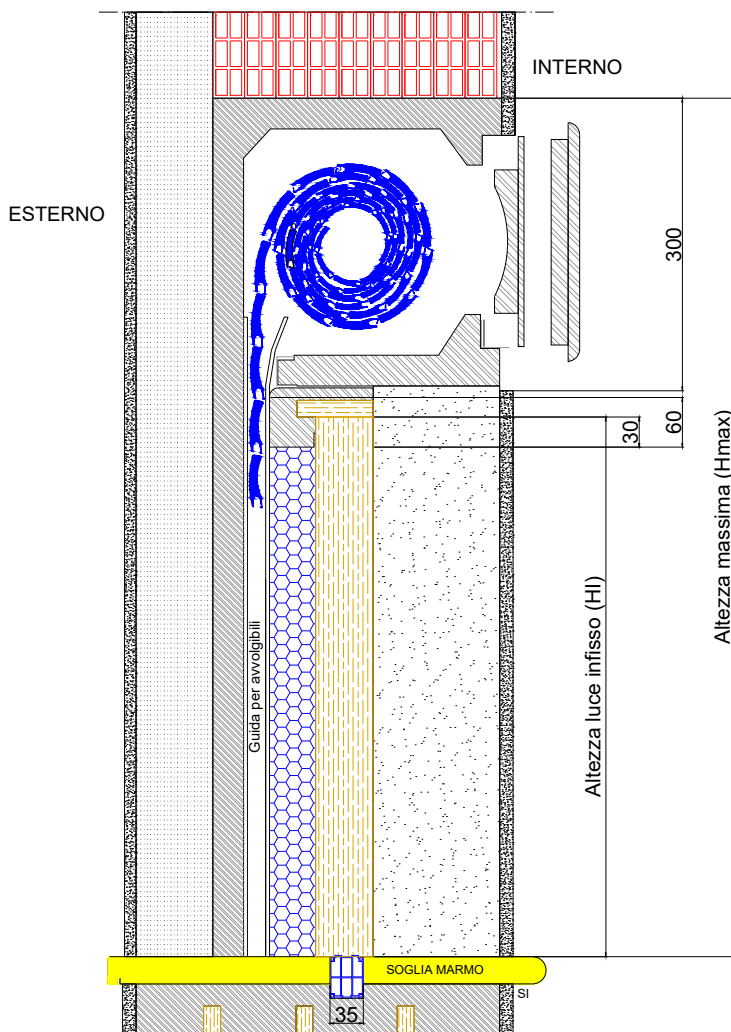
Sezione laterale
