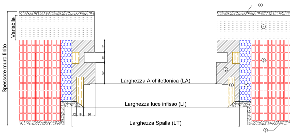
Sezione orizzontale
