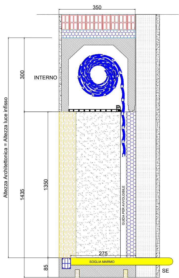
Sezione laterale
