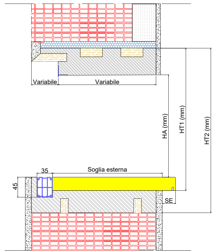
Sezione verticale
