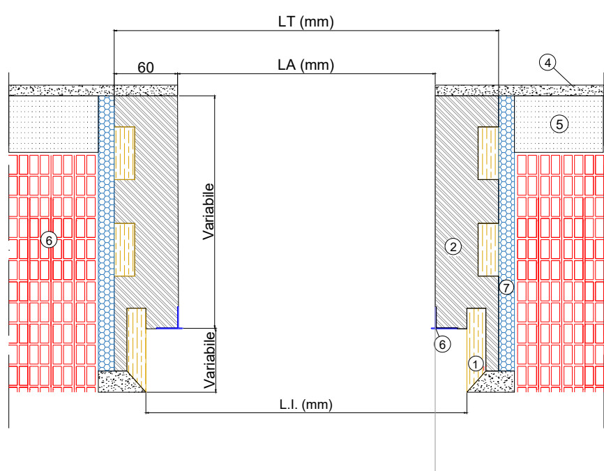
Sezione orizzontale
