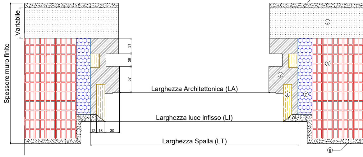
Sezione orizzontale
