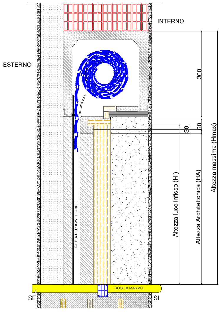
Sezione laterale
